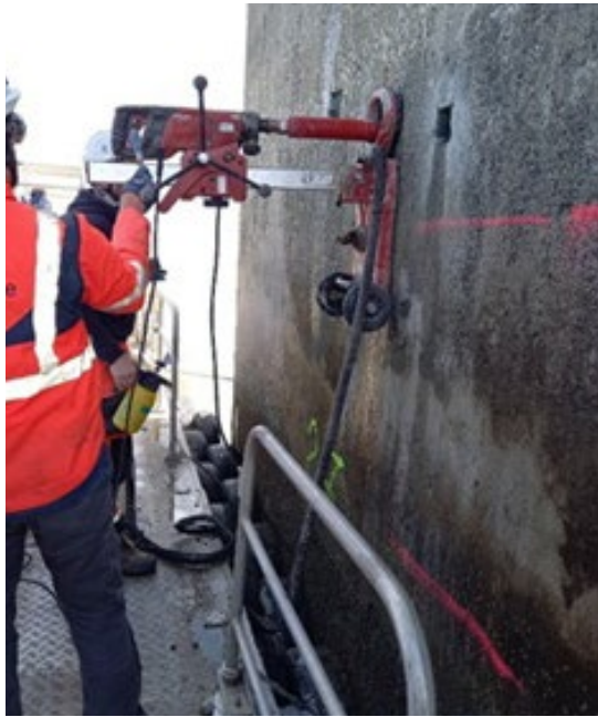
Réalisation de carottages pour analyses béton en labo et création de fenêtre d'autopsie pour vérification du degré de corrosion des armatures
