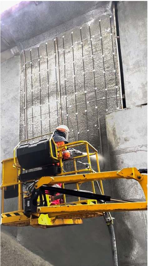
Étape n°3 : Mise en oeuvre du béton projeté
