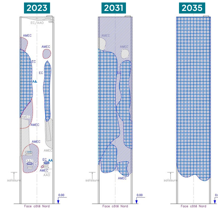
Schémas présentant l'évolution des désordres de la pile 17 (Face Nord) entre 2015 et 2035
