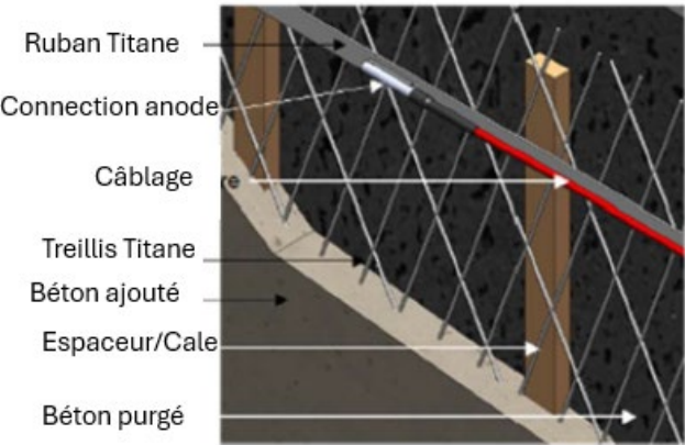
Étape n°2 : Mise en place de la protection cathodique – treillis titane et anodes de connections
